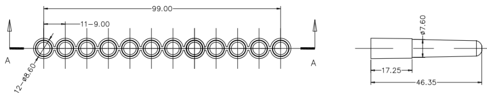
SECTION A-A
